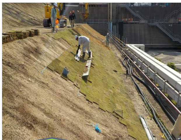
斜面の樹木を伐採し、芝張りをしている作業風景
